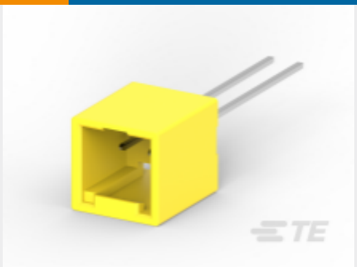
TE 产品编号2-2232546-3 STD 温度信号 GRACE INERTIA 公端
