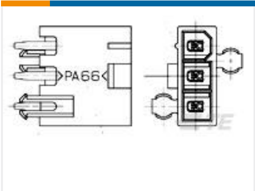
TE 产品编号2029056-5 5P VAL-U-LOK SR HDR SN V0 W/DH
