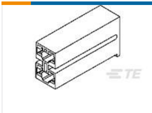
TE 产品编号2-172210-1 PL MKII 187 REC HSG 2P NAT
