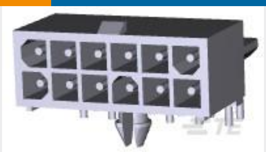
TE 产品编号1-770972-0 12P MINI UMNL R/A HDR ASSY LF
