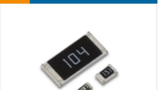
TE 产品编号1-2176347-8 CRGCQ 2010 270R 1%
