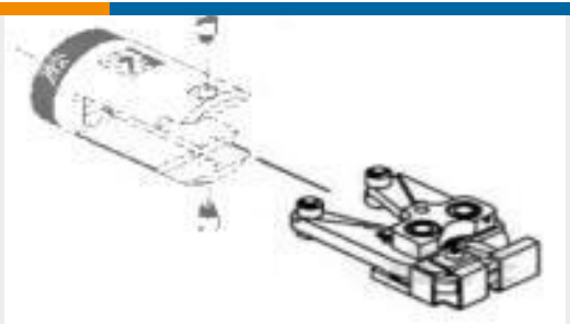
TE 产品编号189896-1 PNEUMATIC CRIMP HEAD 18-8 CES
