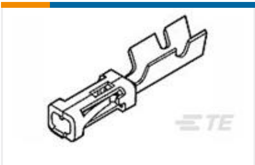
TE 产品编号103455-2 MOD V RECP LP
