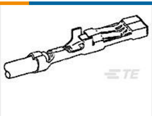
TE 产品编号170286-1 MIC REC CONTACT
