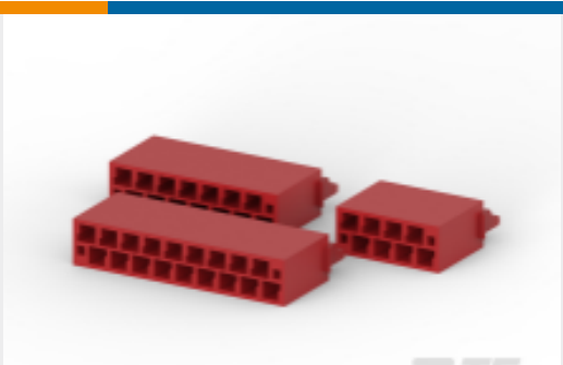
TE 产品编号1-338095-2 扣入式压接外壳
