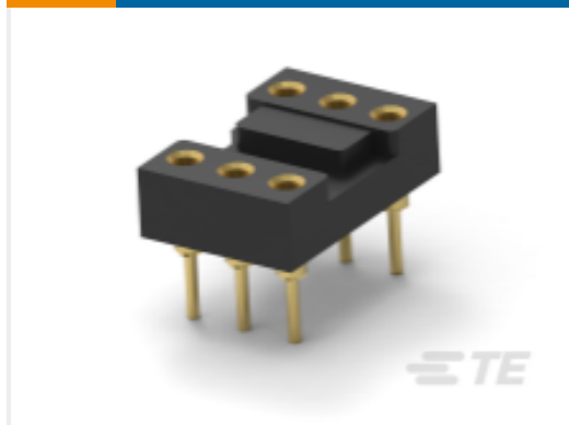
TE 产品编号5-1437536-7 DIP 插座：标准，冲压成型，封闭式，金
