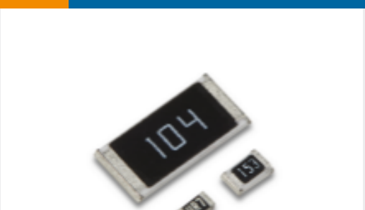
TE 产品编号4-2176345-2 CRGCQ 1210 27K 1%
