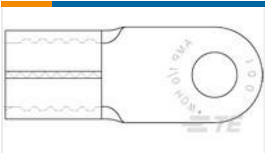
TE 产品编号1958430-1 TERMINAL,STRATO, HR, R, 1/0HD, 5 /16 STUD
