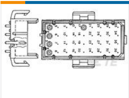
TE 产品编号2-640501-4 09P MR HDR ASSY VO RED LF
