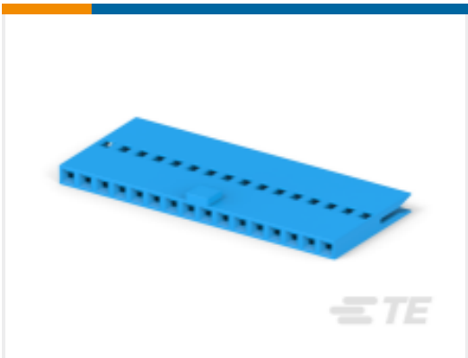
TE 产品编号2-487406-3 2.54mm FFC 连接器母端子
