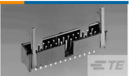
TE 产品编号1-1761609-5 IDC LOW PRO HDR 50P RA SHT LAT
