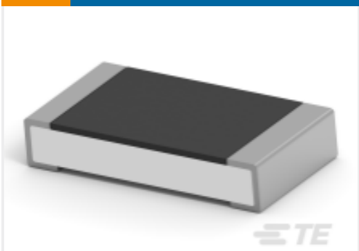
TE 产品编号1-2176390-5 RQ 1206 1K62 0.1% 10PPM 5K RL
