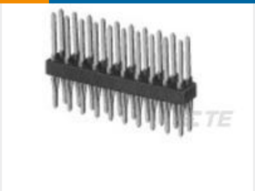
TE 产品编号1-103233-9 40 MODII HDR DRST UNSHRD A/PIN
