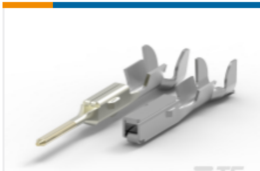
TE 产品编号1376700-1 MULTILOCK，母端和公端
