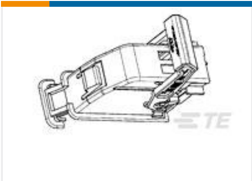
TE 产品编号284360-2 18 POS. FRAME ASSY FOR MQS CON
