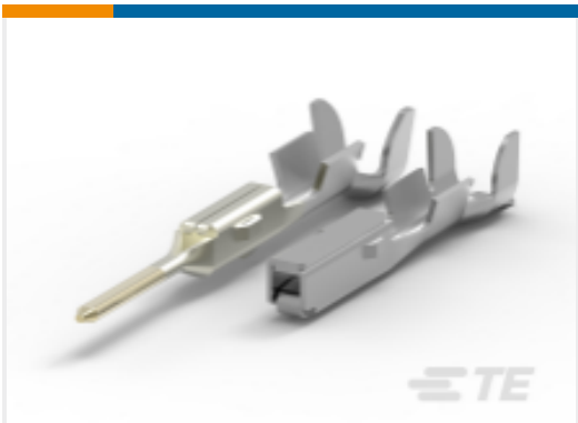
TE 产品编号2109005-2 MULTILOCK，母端和公端
