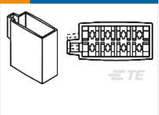
TE 产品编号106455-3 FF 110 PLUG HSG 8P.
