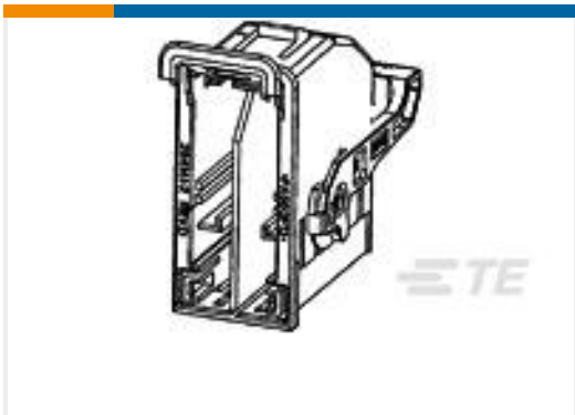
TE 产品编号1745017-1 FRAME 9+9 POS. ASSY
