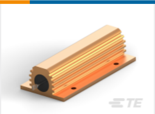
TE 产品编号2-1625999-5 功率电阻器：铝壳体，HSC
