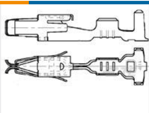
TE 产品编号185026-1 JPT F REC 2.8 Contact SWS Sn
