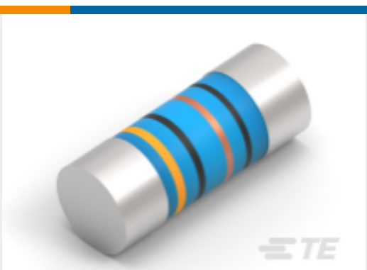
TE 产品编号1-2176315-3 MELF SMA_A 1K0 0.1% 15PPM 0204 0.4W
