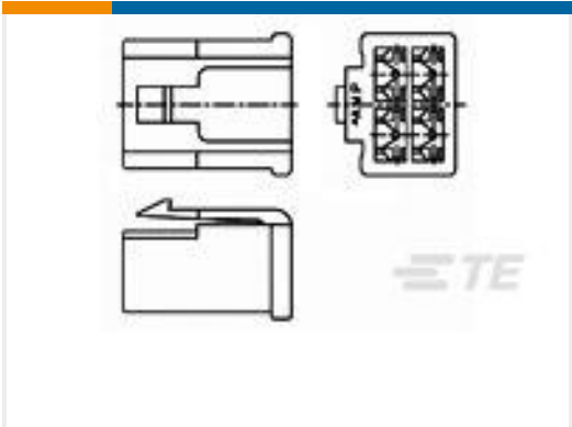
TE 产品编号174202-1 250 FASTON HSG.,REC.,4 POS, NATURAL
