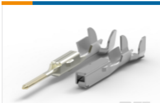
TE 产品编号175276-2 MULTILOCK, 母端和公端
