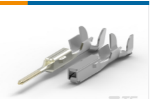
TE 产品编号179967-2 MULTILOCK，母端和公端
