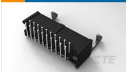
TE 产品编号2-1761607-3 IDC LOW PRO HDR 10P RA LG LAT
