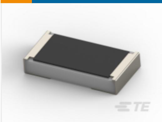
TE 产品编号2176230-5 SMD 功率电阻器：3 瓦特，1% Tol
