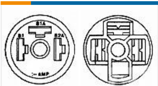
TE 产品编号626311 FASTIN-ON REC.HSG
