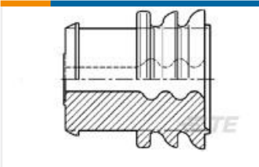
TE 产品编号963245-1 EINZELLEIT-DICHTUNG
