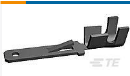
TE 产品编号160859-2 FF 250 TAB 0.5-1.0MM2 TPBR
