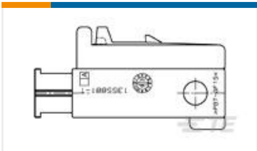
TE 产品编号1355881-1 MQS GRIFFSCHALE 6P
