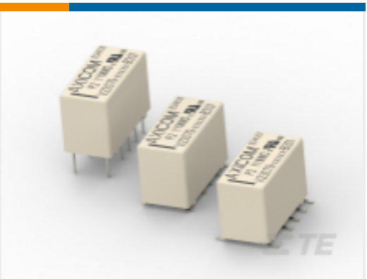
TE 产品编号3-1393788-5 AXICOM P2 标准
