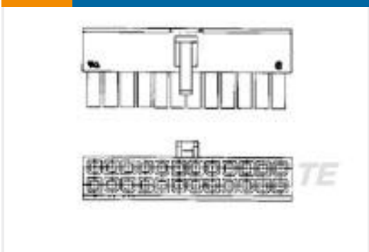
TE 产品编号2-794954-2 22P RCPT VAL-U-LOK V2
