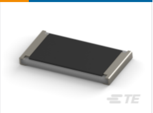
TE 产品编号2176071-8 SMD 功率电阻器：2 瓦特，3521 系列
