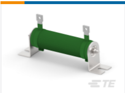
TE 产品编号1879448-4 线绕电阻器：矿物，2.5 Kw
