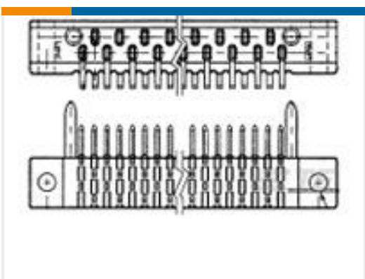
TE 产品编号3-582152-4 35 AMP BLADE HDR ASSY
