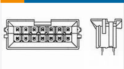
TE 产品编号1586585-4 4P VAL-U-LOK BMI VRT HDR V2
