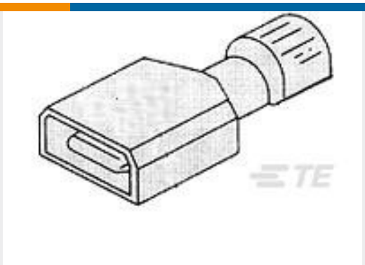
TE 产品编号2-521102-2 ULTRA-FAST 187 ASY Tab 22-18 TPBR
