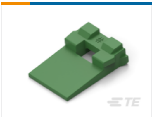
TE 产品编号2600024-1 2CCT ML-XT WEDGELOCK RECEPT GREEN
