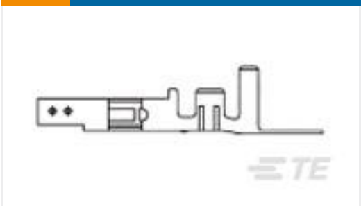
TE 产品编号1586315-1 VAL-U-LOK SKT BR SN 24-18 LP
