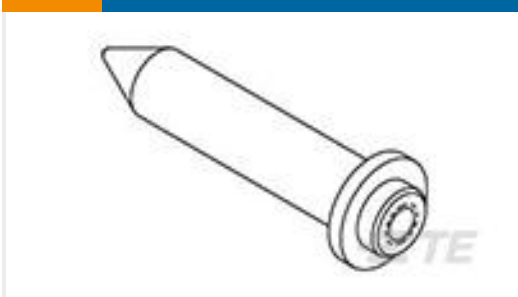
TE 产品编号120985-1 UNV PWR MDL, GUIDE PIN PLTD
