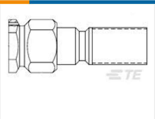
TE 产品编号1051788-1 SMA CABLE PLUG 2031 8052 92
