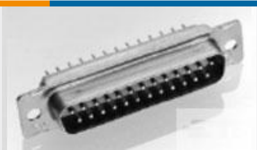
TE 产品编号211669-4 HD 90 44 POS GMT ASY REC HSG
