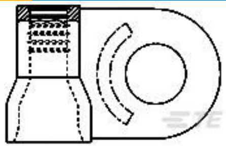
TE 产品编号 32065 TERMINAL,BODY FLAG R 22-16 6
