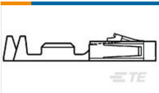
TE 产品编号1658690-1 D-Sub 压接插座，信号，15 针脚，22 号插座，外壳尺寸 1
