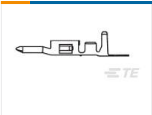
TE 产品编号1586316-3 VAL-U-LOK PIN PHBZ SN 26-22 LP
