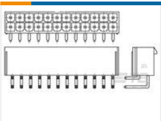
TE 产品编号1-1586041-2 12P VAL-U-LOK R/A HDR V2
