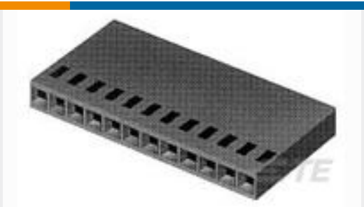
TE 产品编号3-87499-8 20 MODIV HSG COMP SR .100CL
