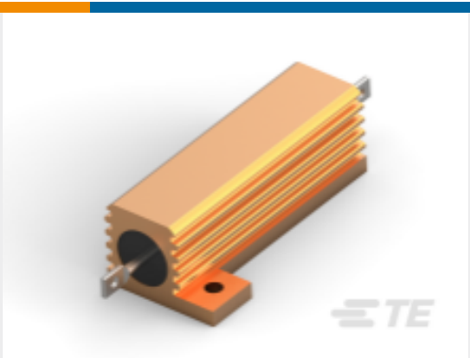
TE 产品编号1676814-7 功率电阻器：铝壳体，HSA
