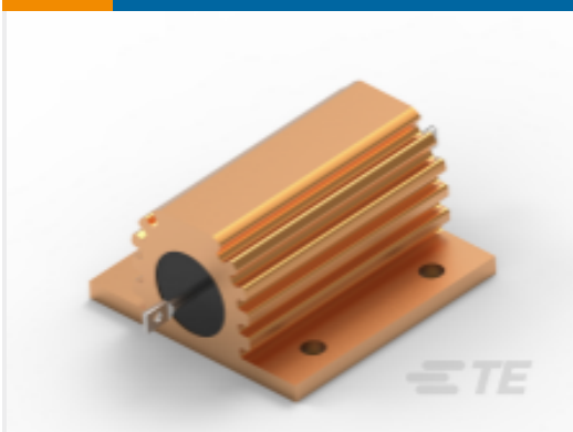
TE 产品编号9-1625984-7 功率电阻器：铝壳体，HSA
