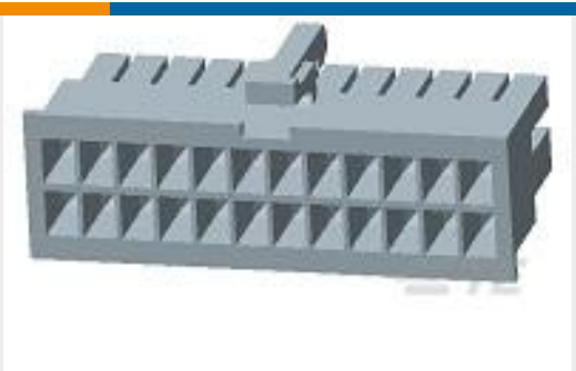
TE 产品编号1969597-6 6P RCPT VAL-U-LOK V2
