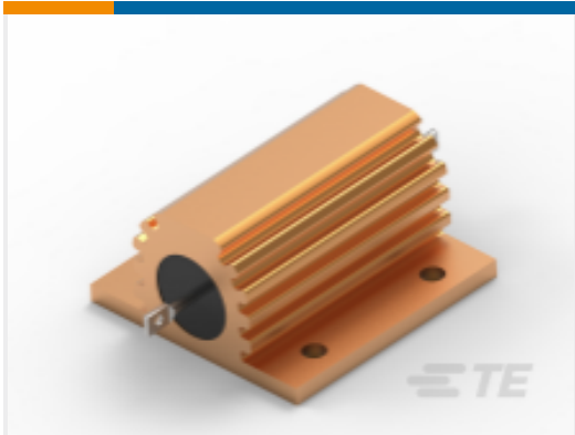
TE 产品编号1625966-8 功率电阻器：铝壳体，HSA
